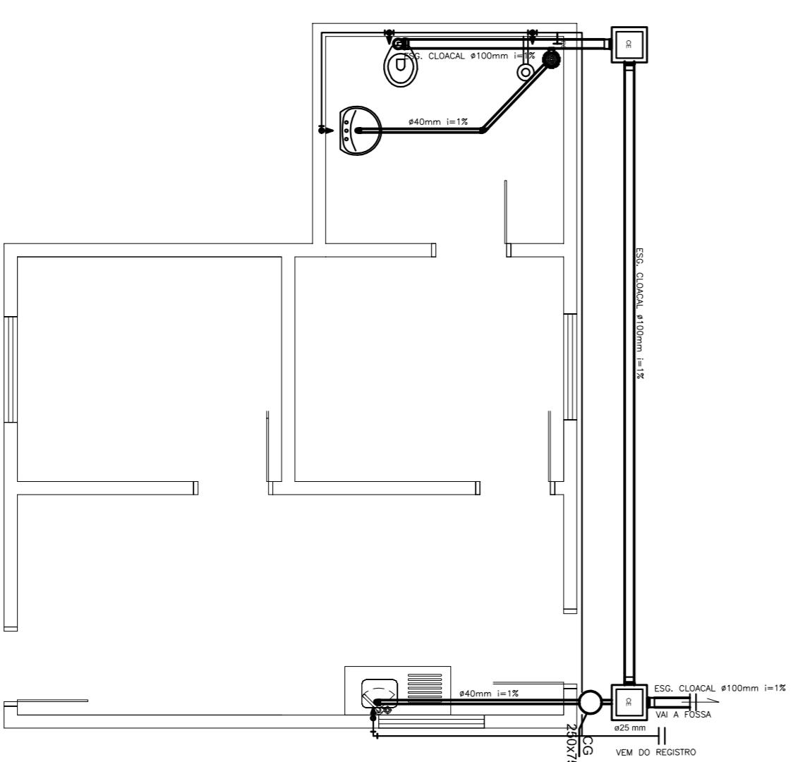
PLANTA BAIXA- CASA ZELADOR
