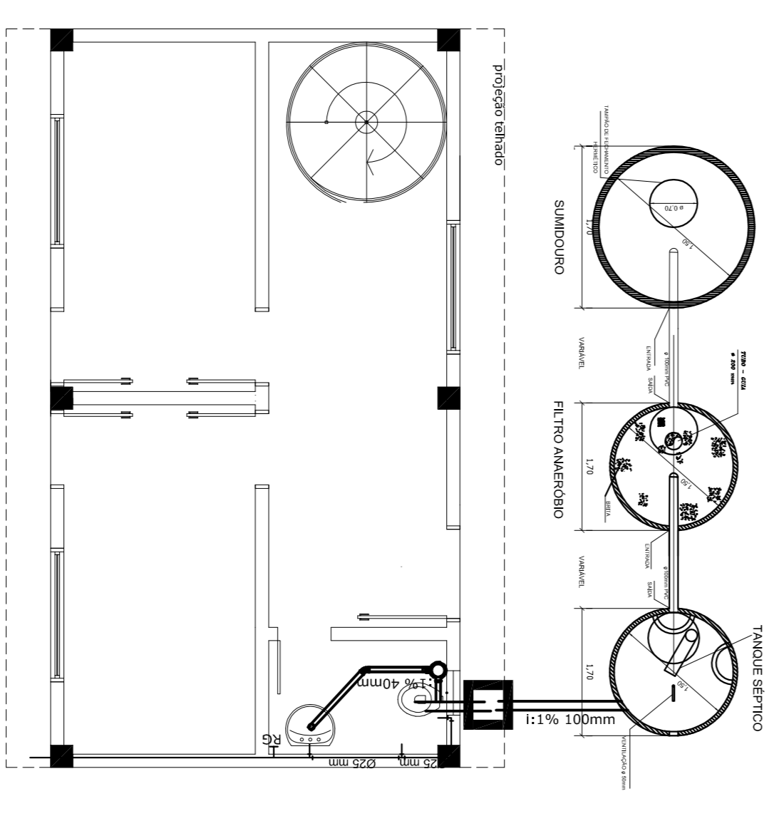
Planta Baixa - pilotis (radialista) E:1/50
